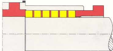
standard stuffing box tenue à presse-étoupe standard
